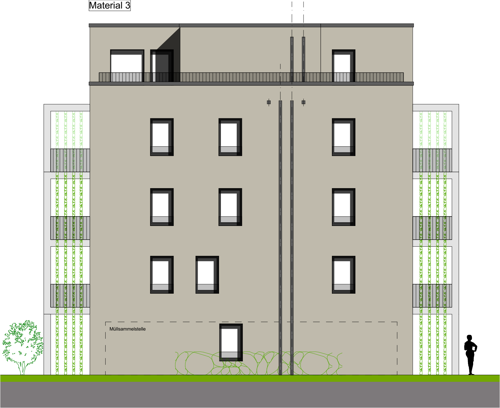
Ansicht Nord-Ost, Seite
